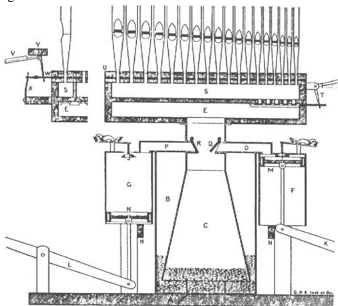
Rys. Organo wodne wg Ktesibiosa (III w.p.n.e.)
